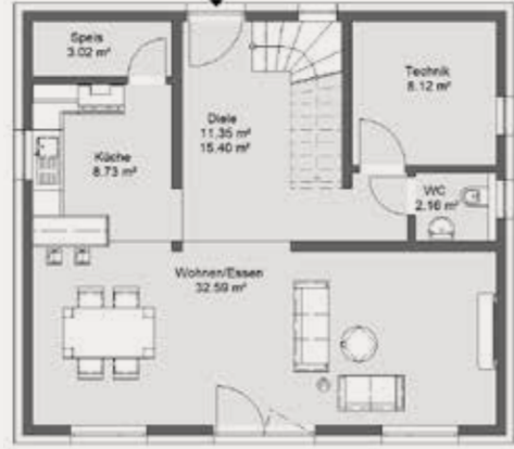
Mit Speis
