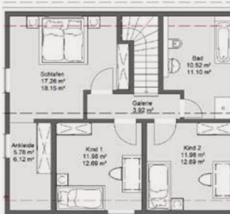
Dachgeschoss Kniestock 180 mit Ankleide
