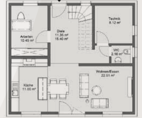
Mit Arbeitszimmer
