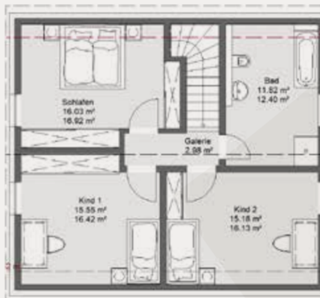
Dachgeschoss Kniestock 180
