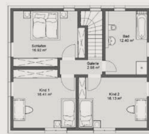
Obergeschoss 2. Vollgeschoss
